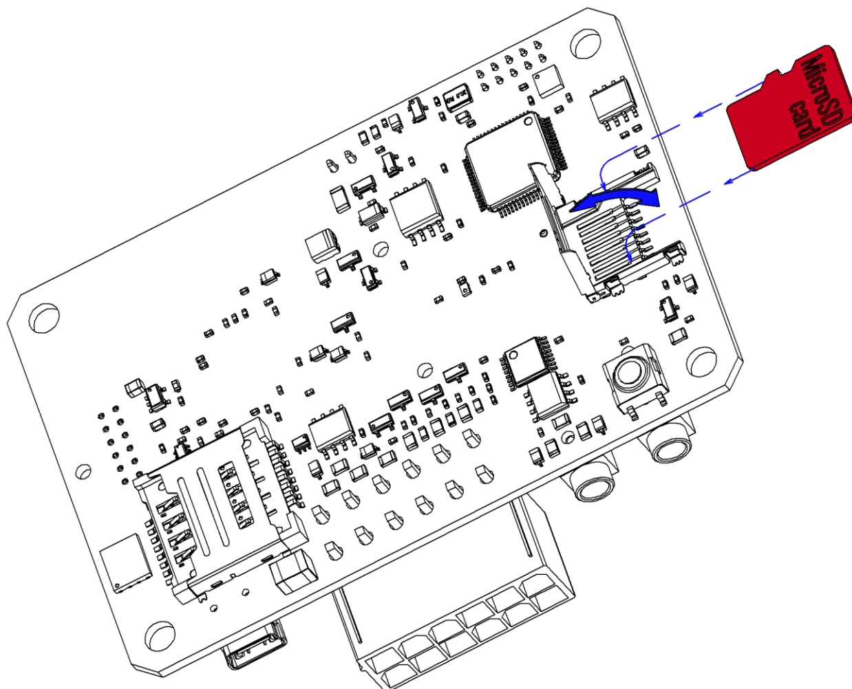
Рисунок 2.10 Установка microSD-карты
