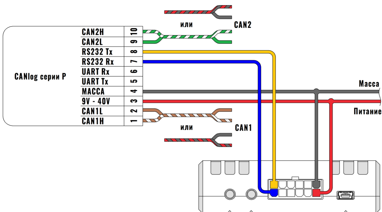
Рисунок 2.27 Подключение CAN-LOG по RS-232
