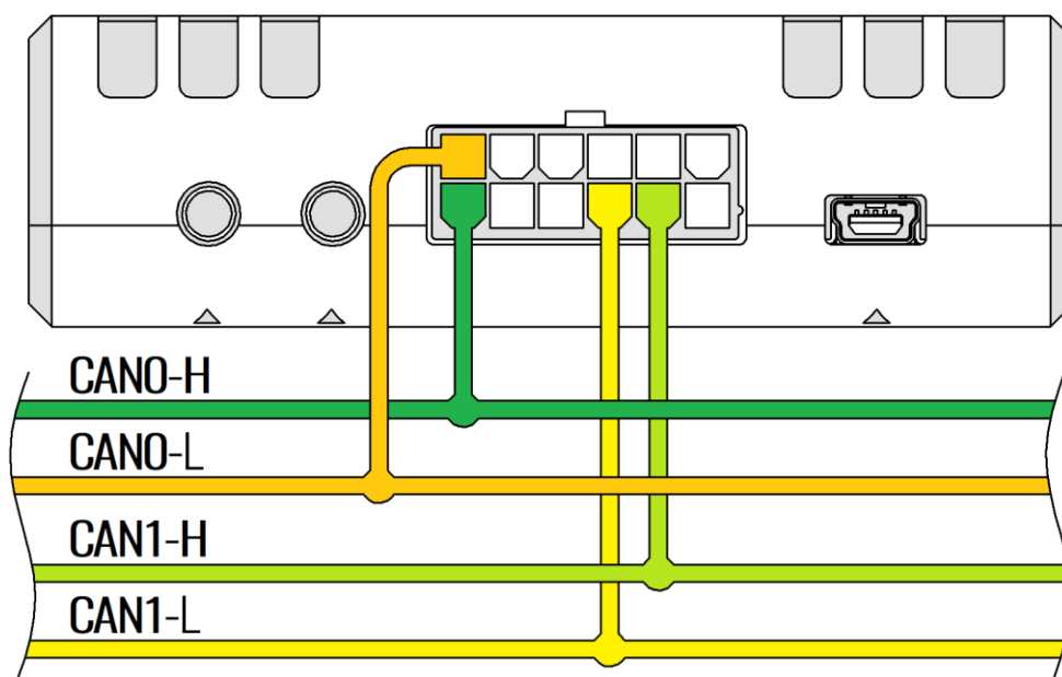
Рисунок 2.24 Подключение к шине CAN
