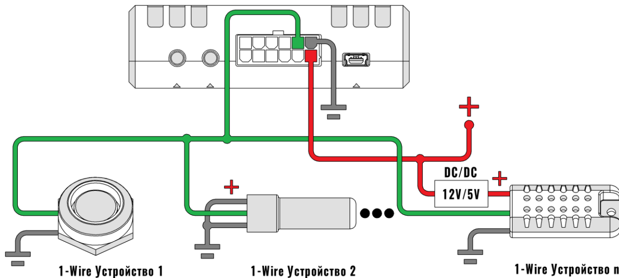
Рисунок 2.26 Подключение устройств по 1-Wire
