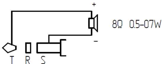
Рисунок 2.29 Схема распайки тангенты
