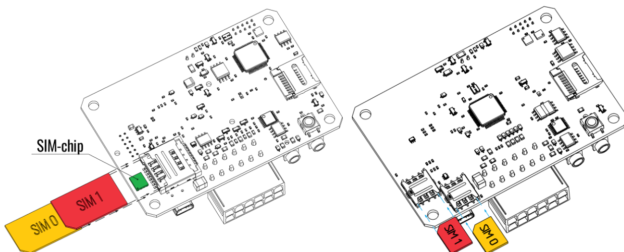
Рисунок 2.8 Установка SIM-карт (справа для УМКа302v2 и УМКа302v3)
