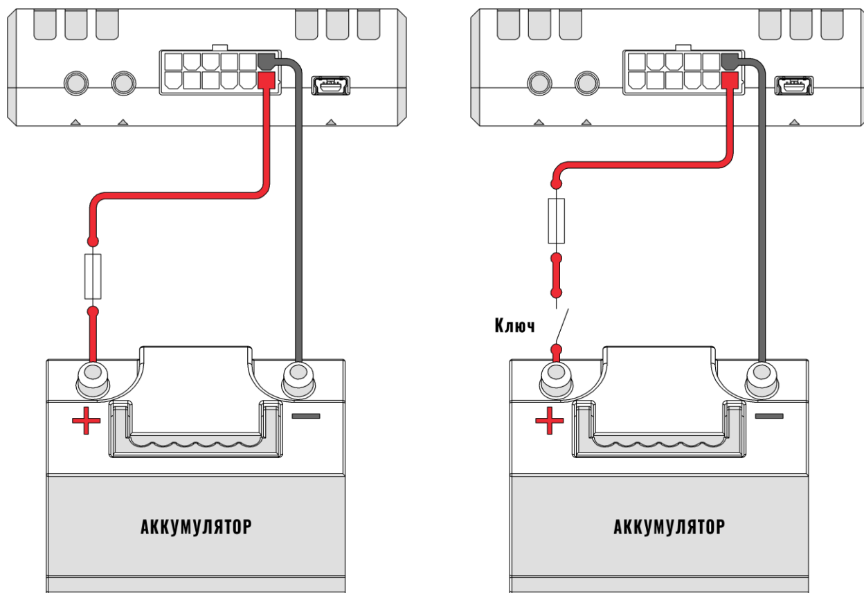
Рисунок 2.11 Подключение питания
