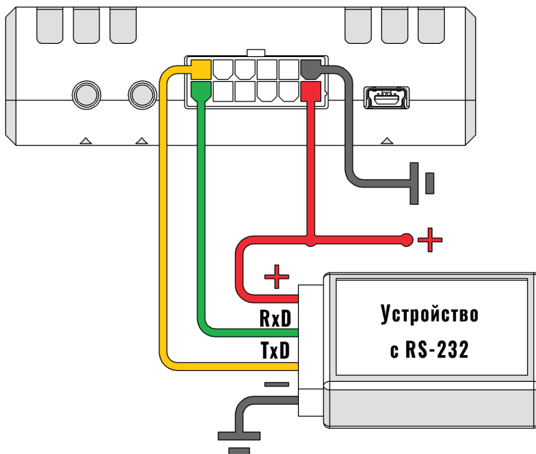
Рисунок 2.25 Подключение по интерфейсу RS-232
