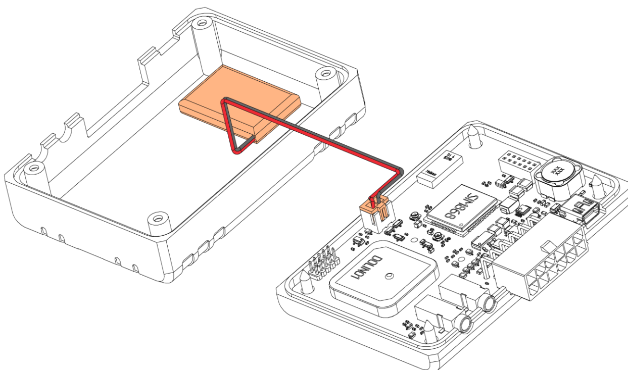
Рисунок 2.9 Установка аккумулятора
