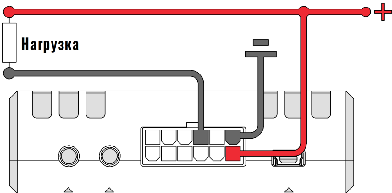
Рисунок 2.19 Подключение маломощной нагрузки
