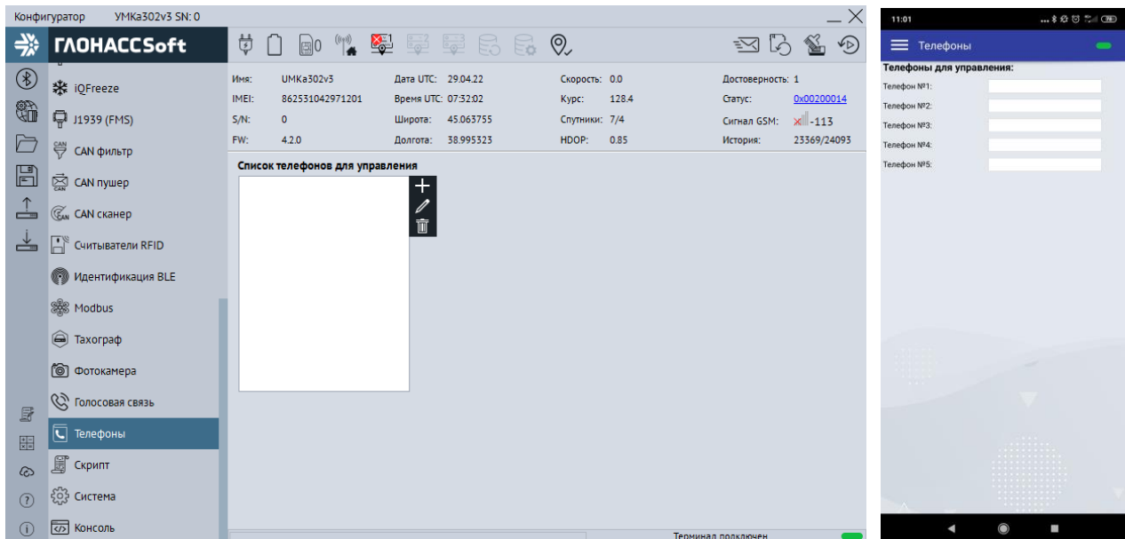
Рисунок 3.45 Вкладка «Телефоны»
