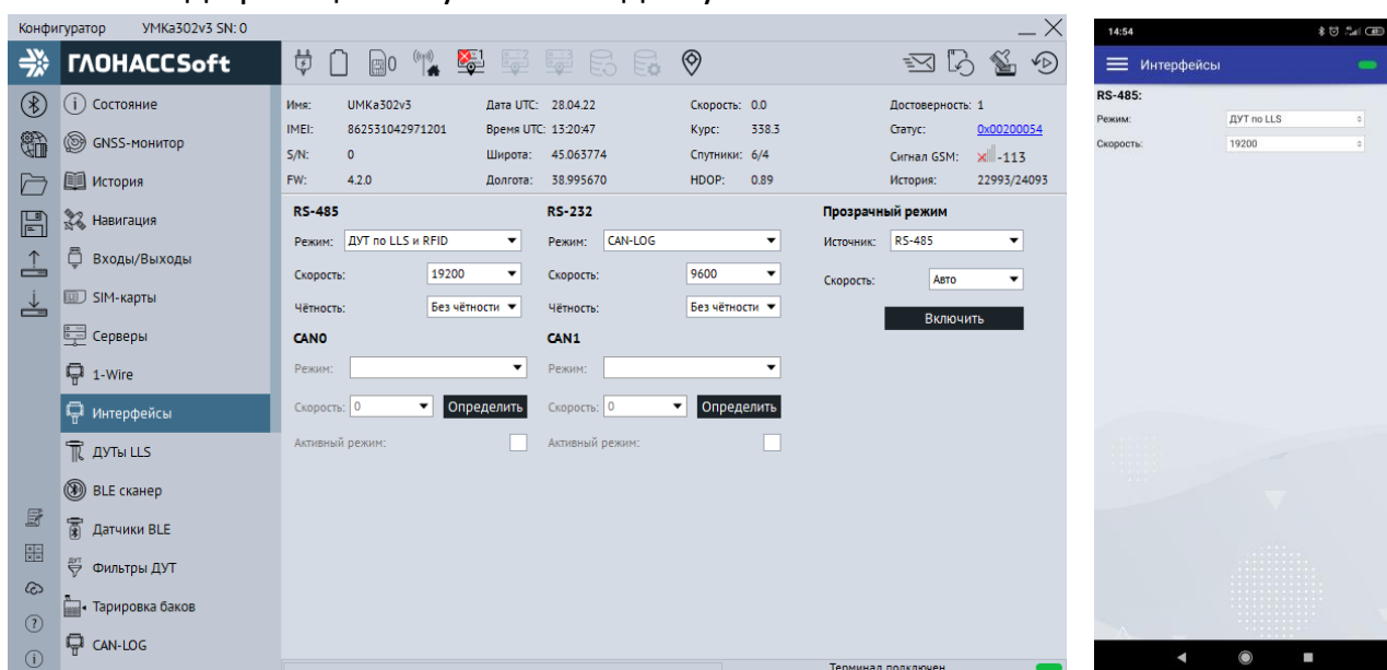
Рисунок 3.23 Вкладка «Интерфейсы»
