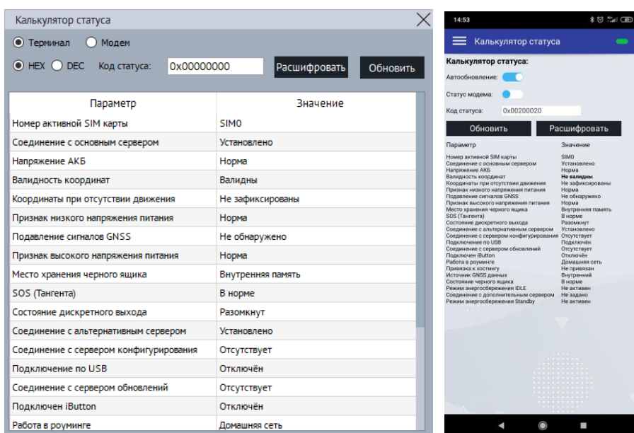
Рисунок 3.14 Калькулятор статуса
