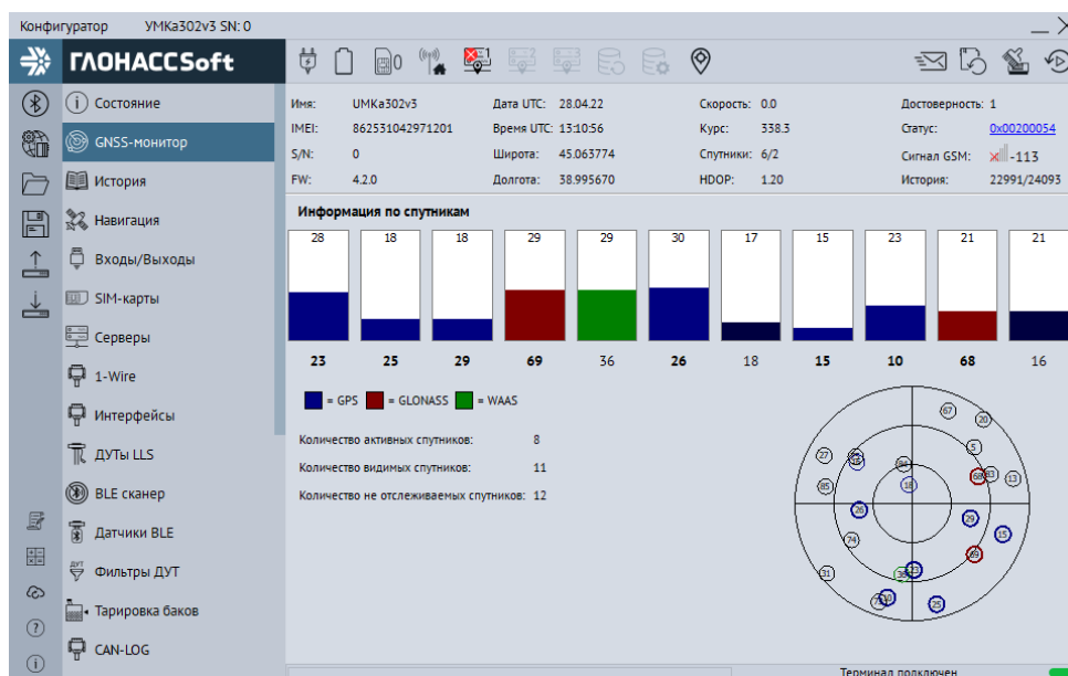
Рисунок 3.15 Вкладка «GNSSS-монитор»
