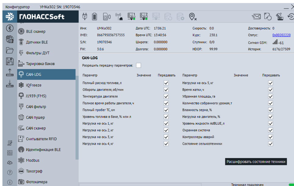
Рисунок 3.30 Вкладка «CAN-LOG»
