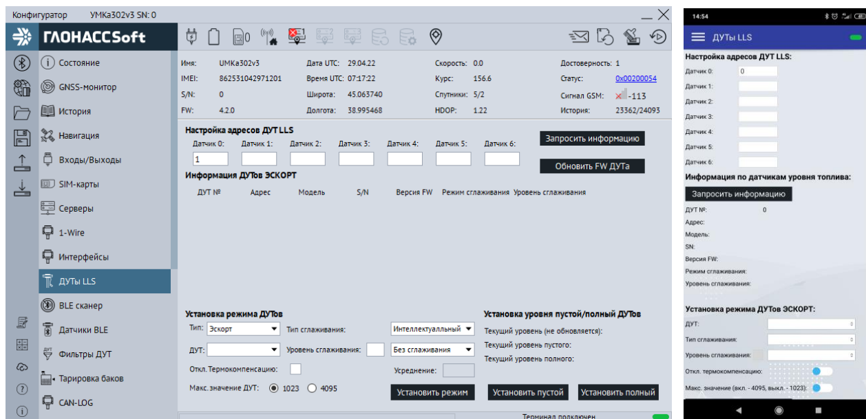
Рисунок 3.24 Вкладка «ДУТы»
