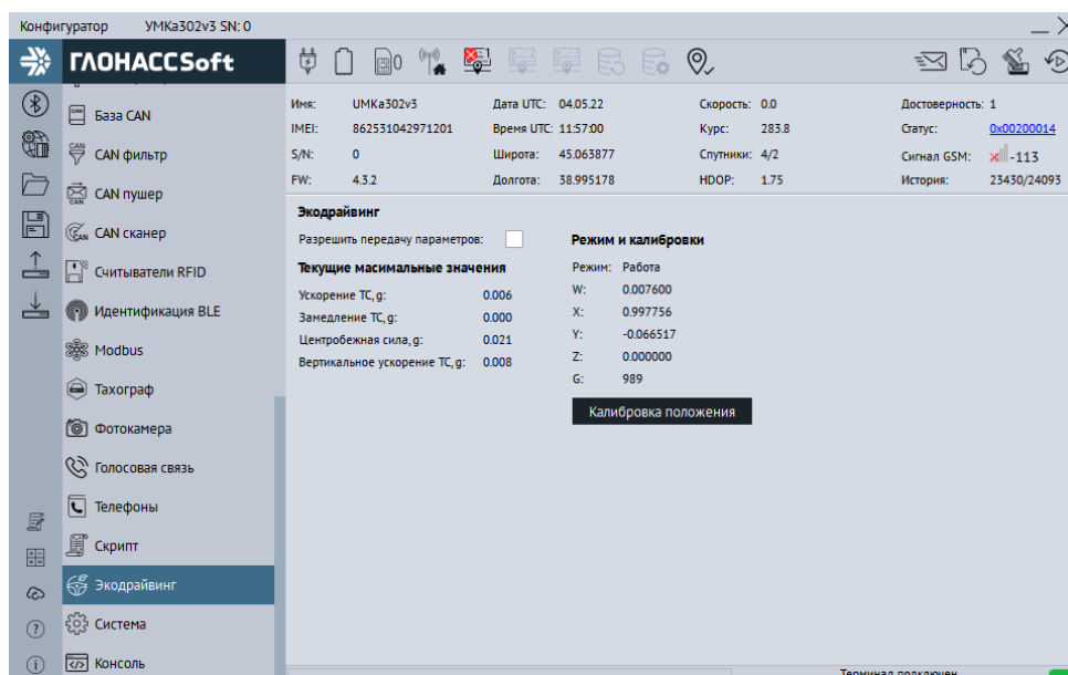
Рисунок 3.50 Вкладка «Экодрайвинг»
