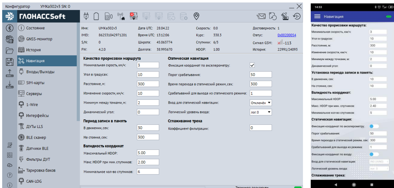
Рисунок 3.17 Вкладка «Навигация»
