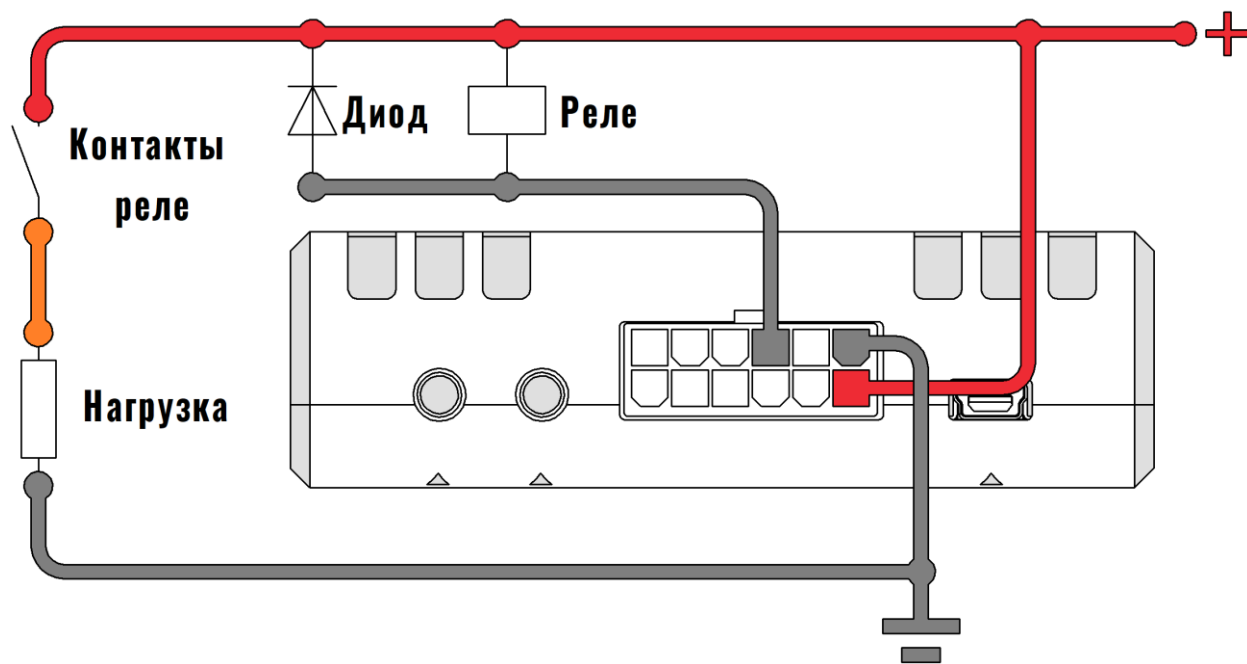
Рисунок 2.20 Подключение мощной нагрузки
