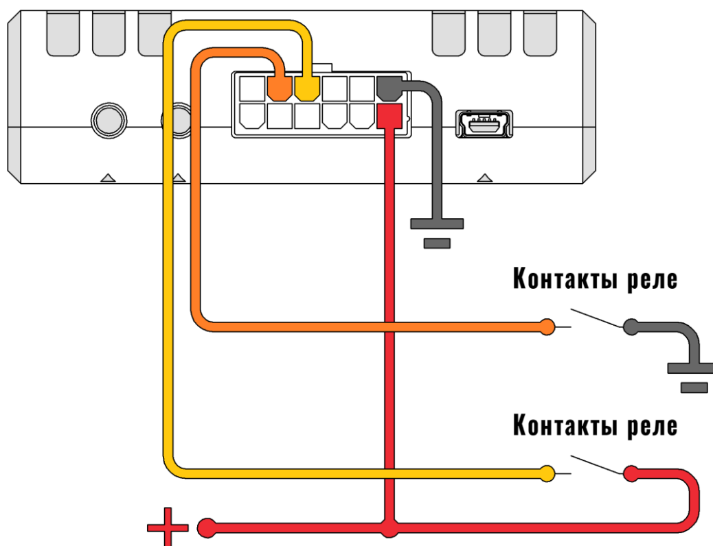
Рисунок 2.16 Варианты подключения дискретных датчиков
