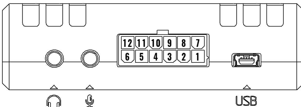
Рисунок 2.6 Нумерация выводов терминала
