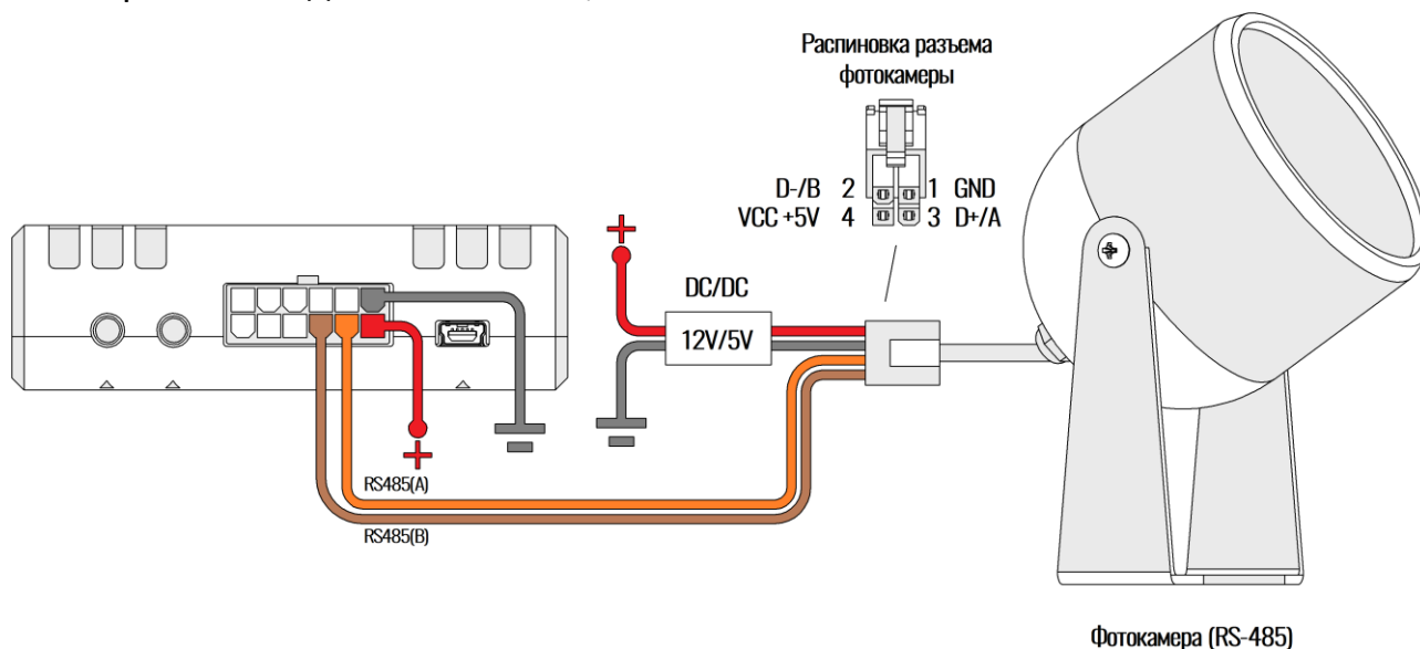
Рисунок 2.31 Подключение фотокамеры JC426F-Q01 с RS-485
