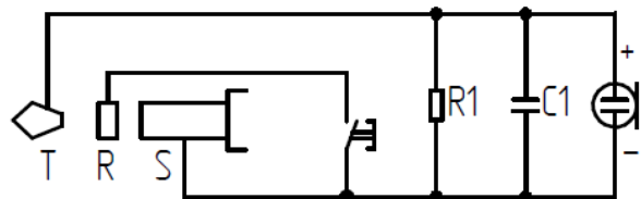
Рисунок 2.29 Схема распайки тангенты
