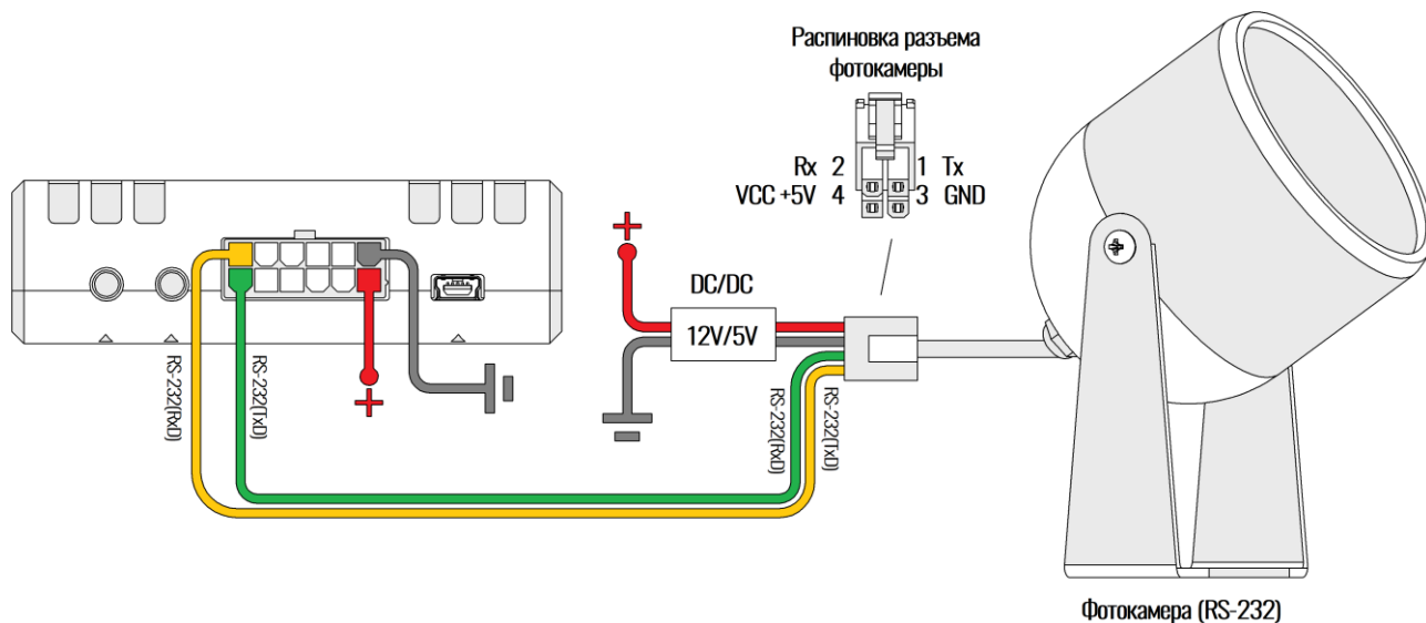
Рисунок 2.30 Подключение фотокамеры JC029F-Y01 с RS-232
