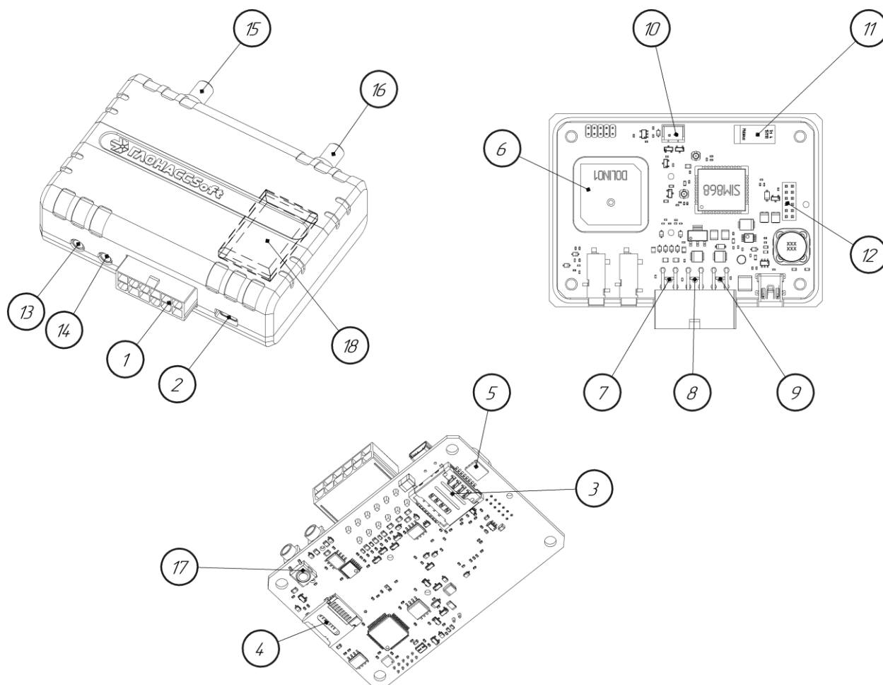
Рисунок 2.5 Основные элементы терминала
