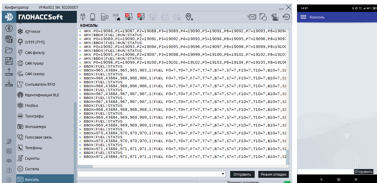
Рисунок 3.53 Вкладка «Консоль»
