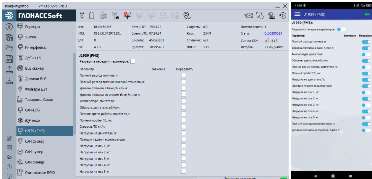
Рисунок 3.33 Вкладка «J1939(FMS)»
