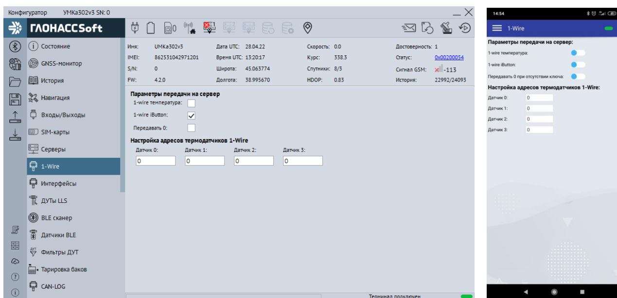
Рисунок 3.22 Вкладка «1-Wire»
