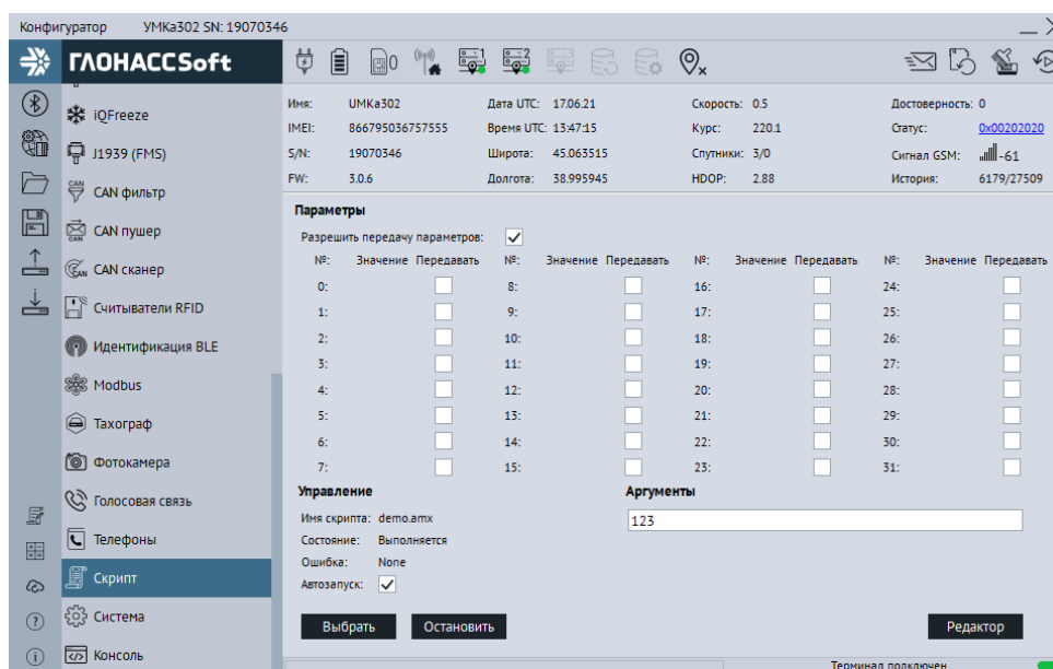
Рисунок 3.48 Вкладка «Скрипты»
