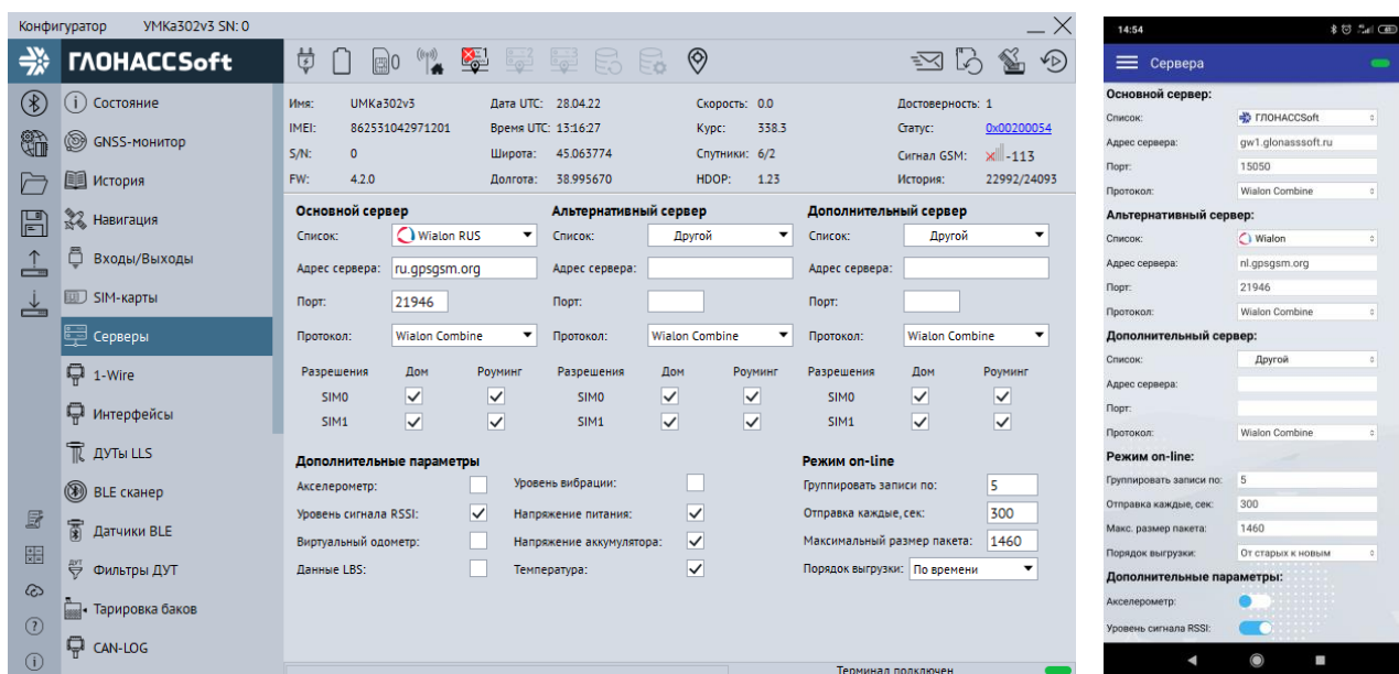
Рисунок 3.21 Вкладка «Серверы»
