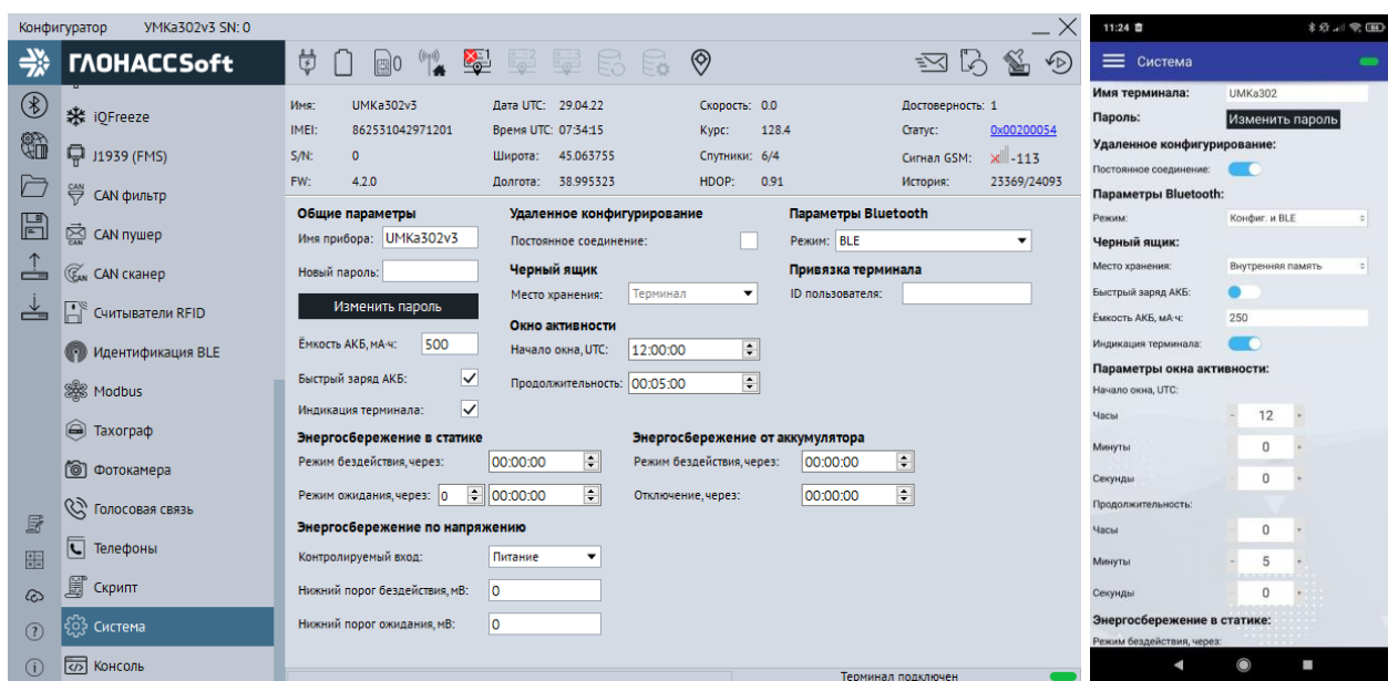
Рисунок 3.52 Вкладка «Система»
