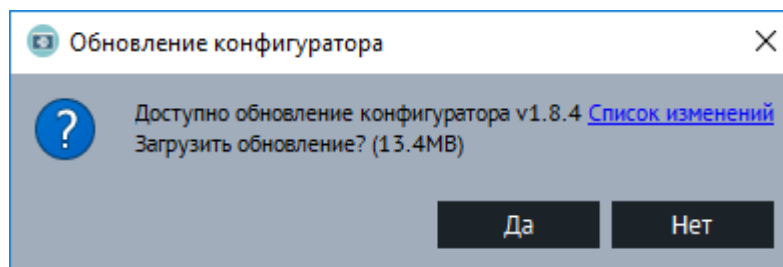
Рисунок 3.9 Обновление конфигулятора
