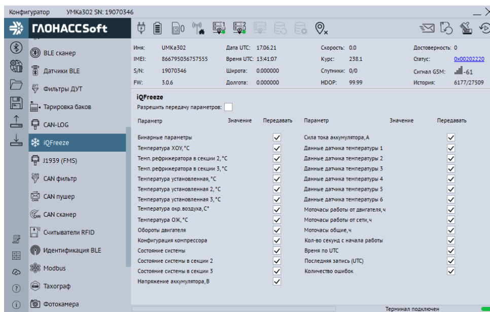
Рисунок 3.32 Вкладка «iQFreeze»
