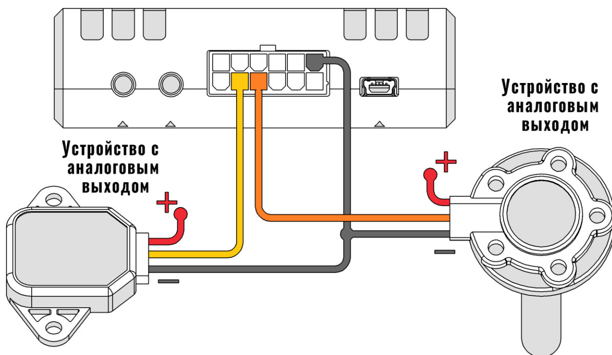
Рисунок 2.12 Подключение аналоговых источников
