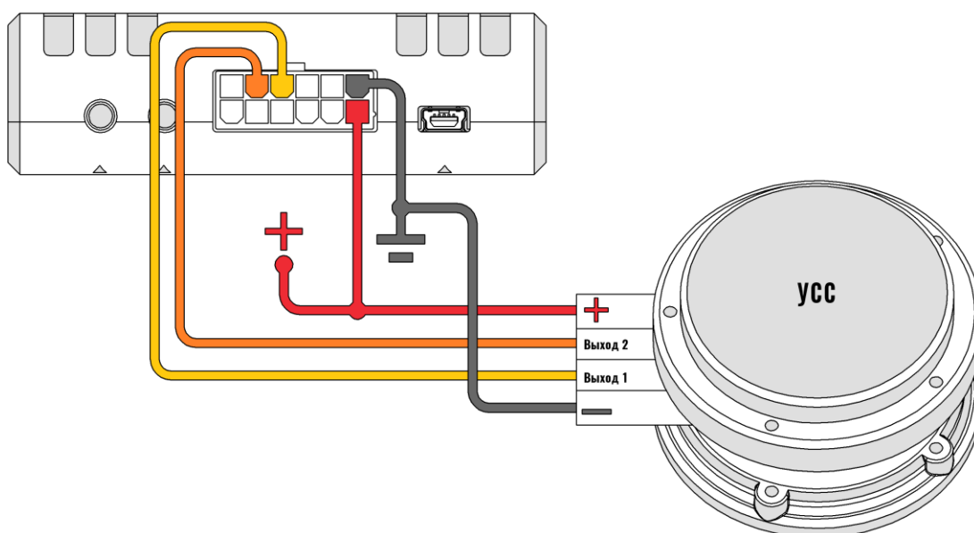
Рисунок 2.18 Пример подключения УСС
